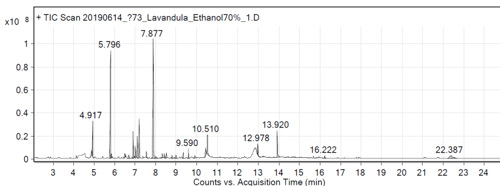
Рис.1.Хроматограмма настойки надземных органов Lavandula angustifolia Mill.
